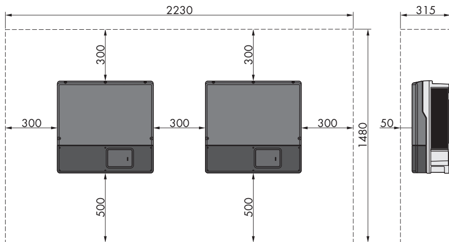
図 5: 推奨間隔 (mm単位 of 寸法)
