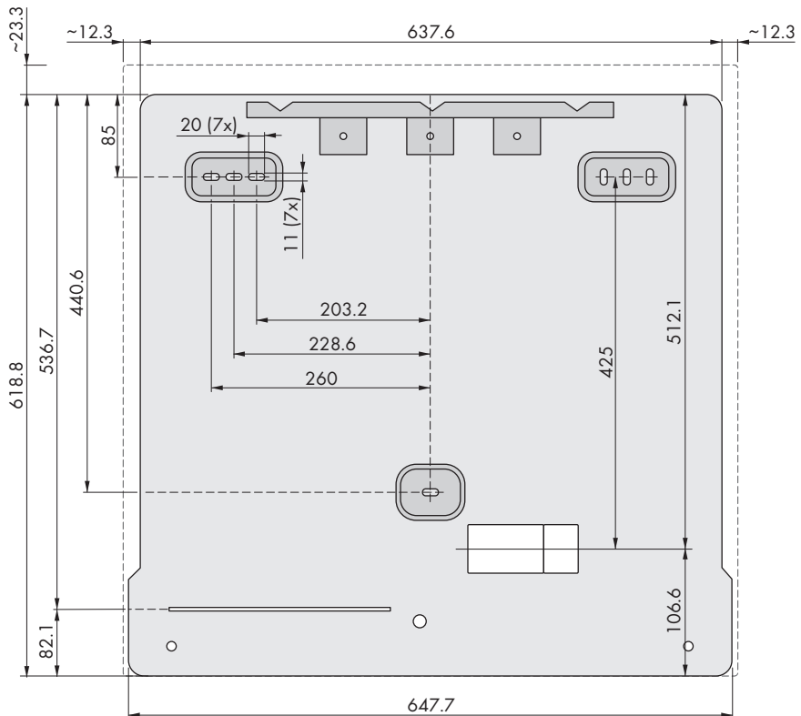
図 4: 取付穴の位置（寸法の単位：mm）
