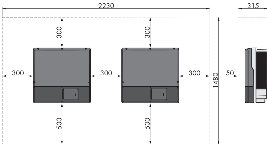
図 5: 推奨間隔 (寸法の単位: mm)
