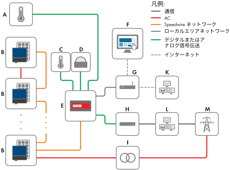
図 2: Cluster Controller 装備の大規模な分散型発電システム、ならびに開ループ制御による電力会社制値の実装 (例)
