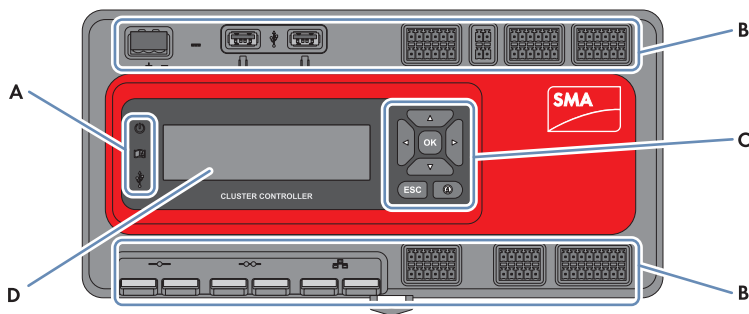
図 1: Cluster Controller の前面
