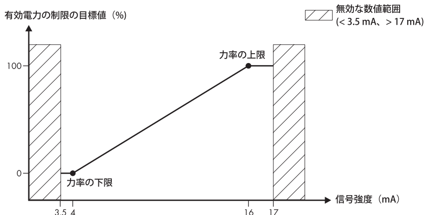
図 8: パワーコンディショナの設定した有効電力限界（Pmax）パラメータで設定される制値の上限と下限（例）
