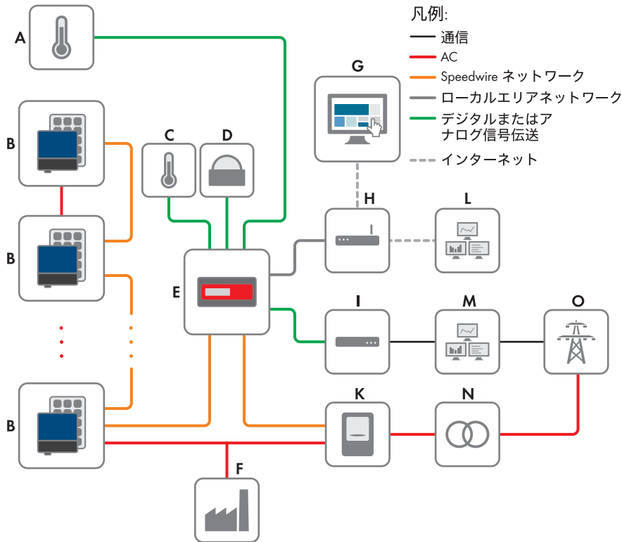
図 3: Cluster Controller 装備の大規模な分散型発電システム、ならびに閉ループ制御による電力会社制御値の実装 (例)
